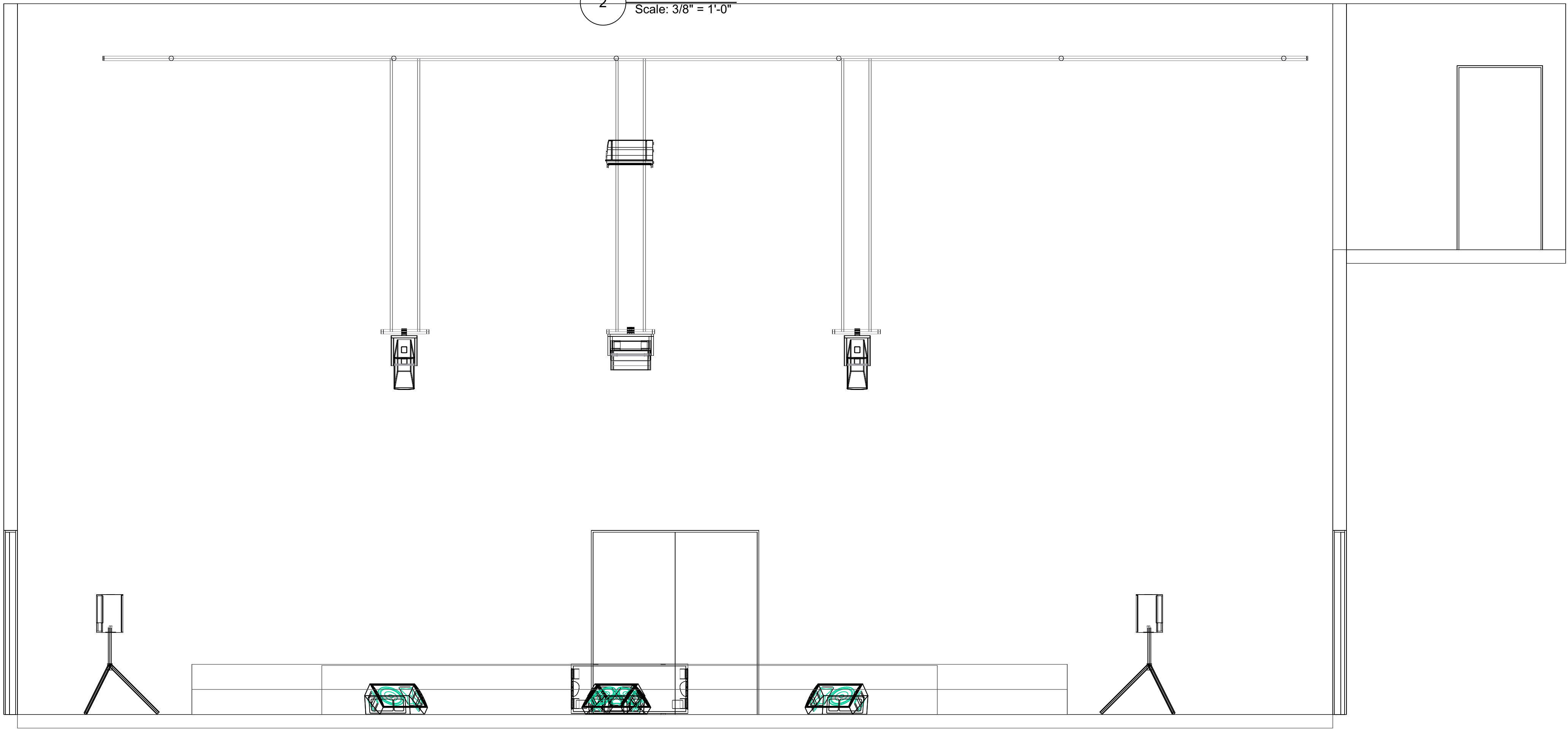
3 Section Scale: 3/8" = 1'-0"
